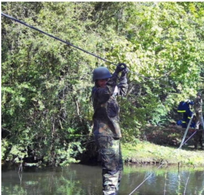
Seilsteg
